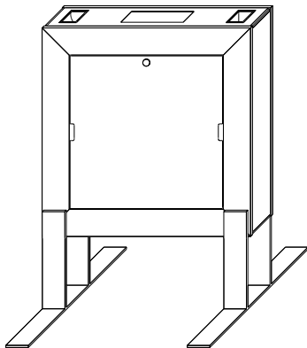
ENERCON Box mit hohem Fußausleger 600 x 810 x 90 mm
